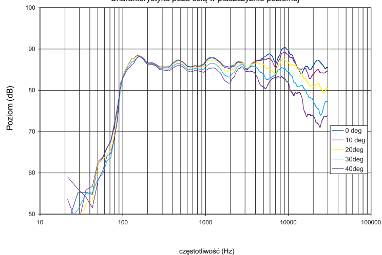
Charakterystyka poza osią w płaszczyźnie poziomej
